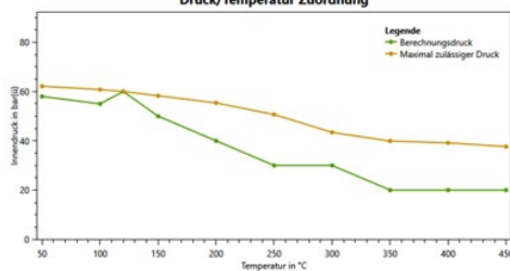
Druck/Temperatur Zuordnung
