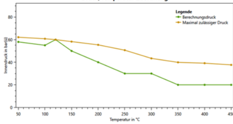
Druck/Temperatur Zuordnung
